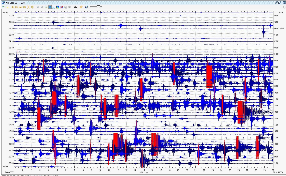
Şekil 1. Santorini-Ege Denizi Deprem Fırtınası 24 saatlik görüntüsü.
