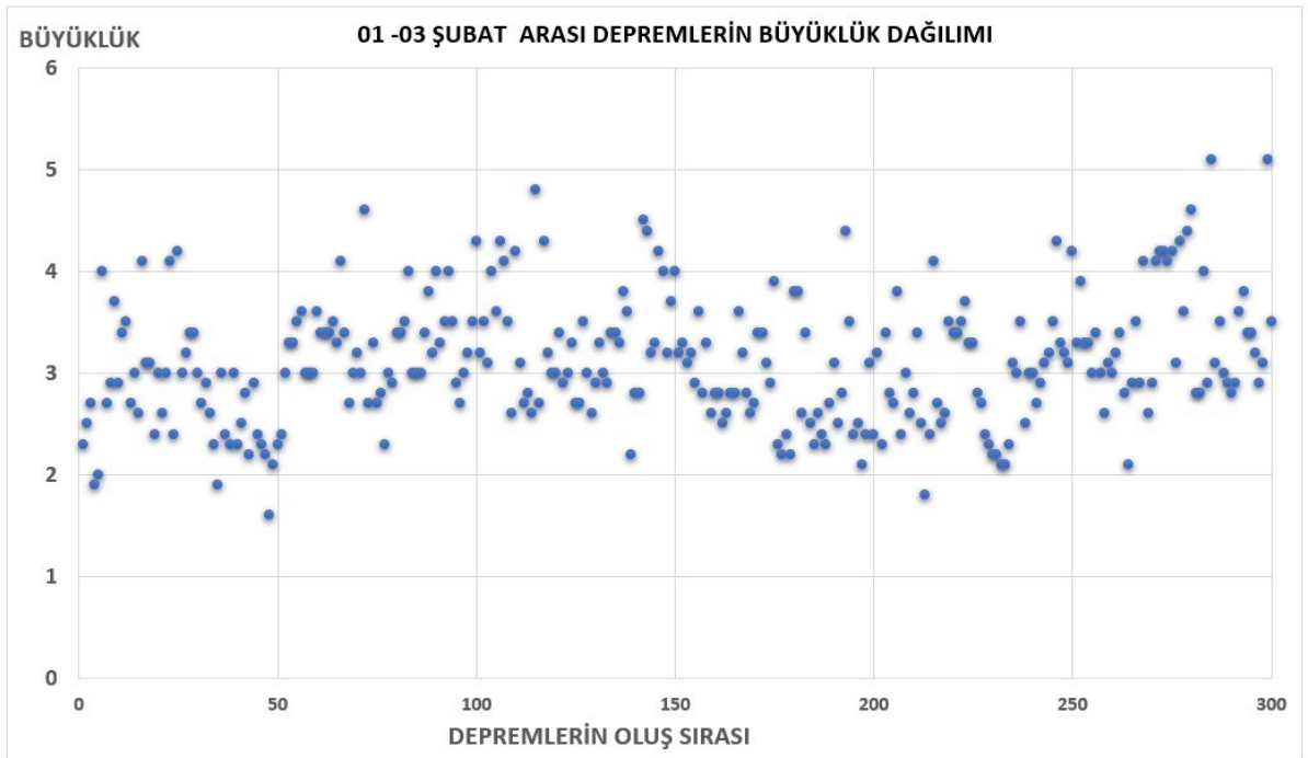
Şekil 3. Santorini- Ege denizi Depremlerinin Büyüklük Dağılımı
