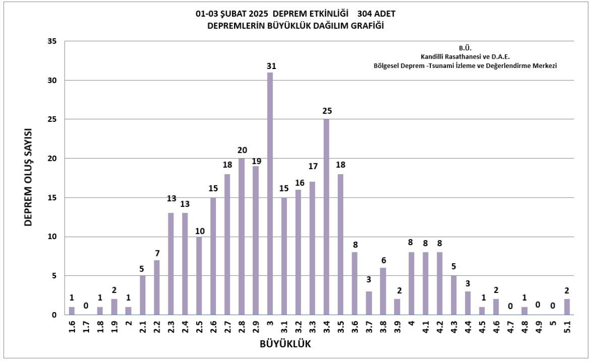
Şekil 4. Santorini- Ege denizi Depremlerinin Büyüklük Dağılımı
