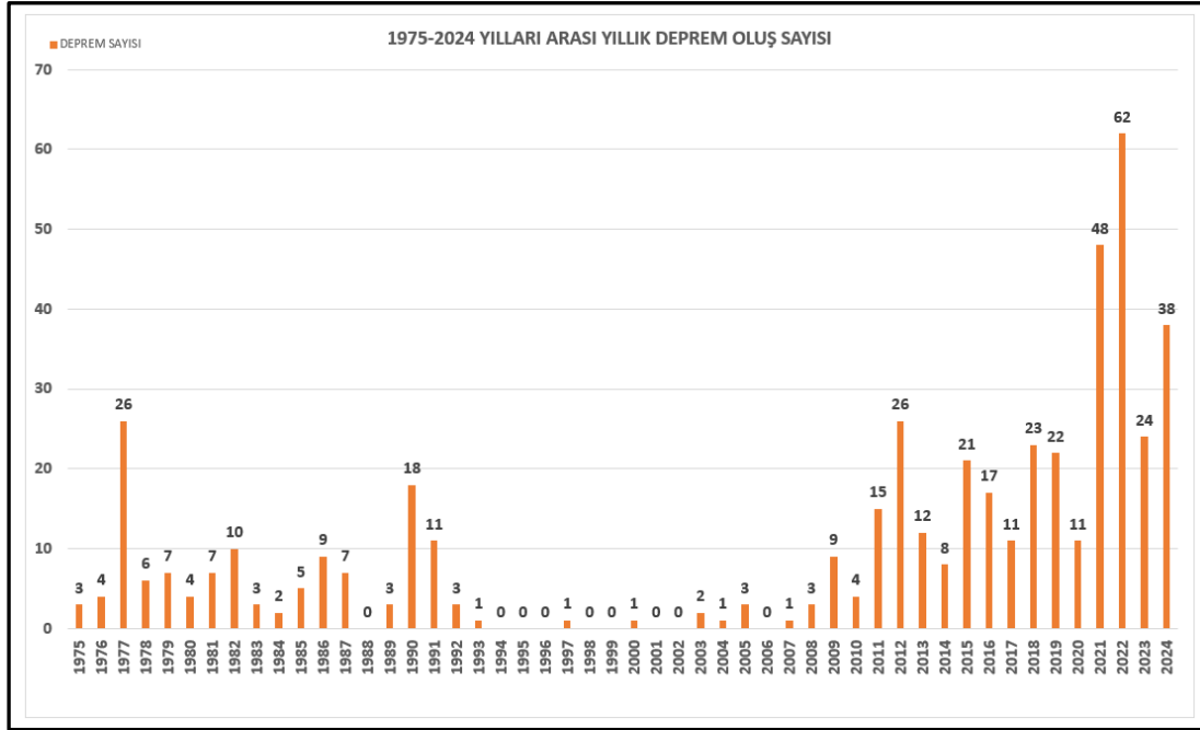
Şekil 7. 1975-2024 Yılları Arası Deprem Oluş Sayısı (1975-2024).
