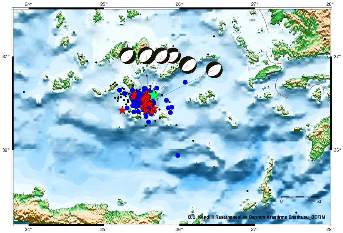
Şekil 2. 31.01.2025-03.02.2025 tarihleri arası bölgenin deprem etkinliği ve odak mekanizması çözümleri.
