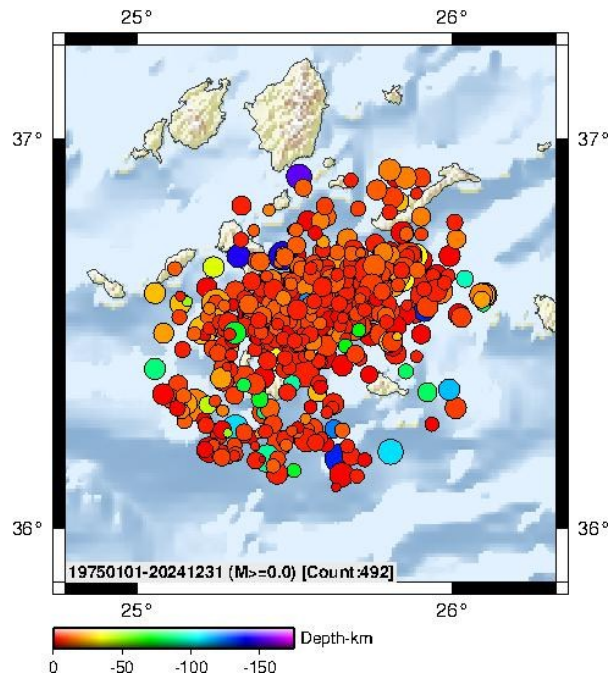
Şekil 5. Bölgenin son 50 yıllık deprem etkinliği.
