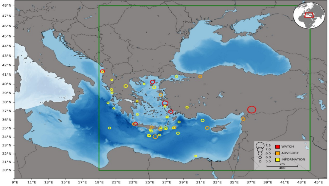
Şekil 8. KRDAE tsunami gözlem alanında Tsunami uyarı mesajı yayınlanan depremler.
