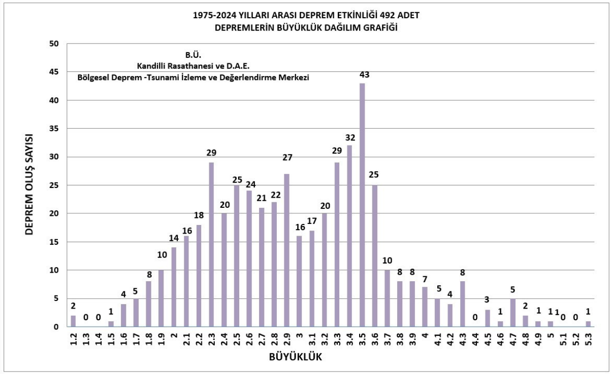
Şekil 6. Deprem-Büyüklik Dağılımı (1975-2024).
